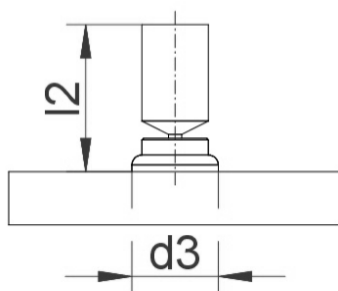
Geschweißter Bolzen
